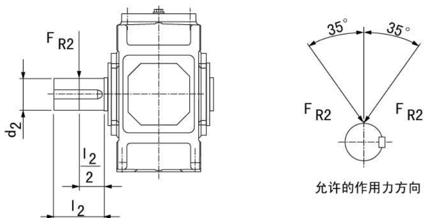
允许的附加径向力 F_{R2} (kN)，作用于输出轴端中部**
