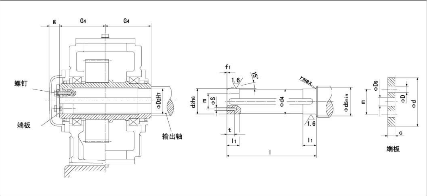
2、带平键联接的空心轴尺寸图表:
