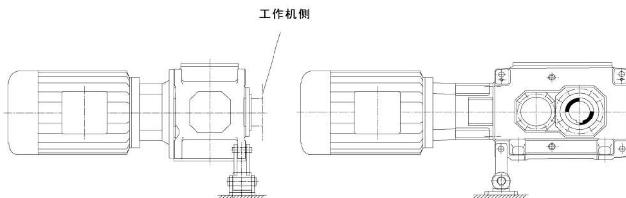
扭力臂式安装
